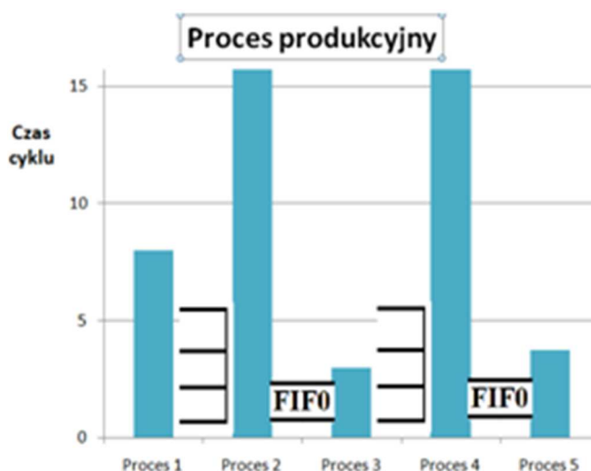
Rys. 2.10. Przykład zastosowania kolejki FIFO pomiędzy procesami o różnych długościach cyklu
