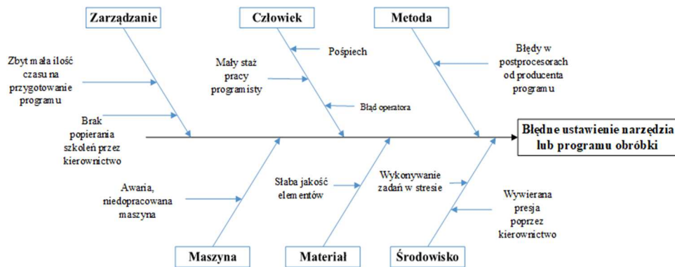
Rys. P15.1. Diagram Ishikawy dla problemu: błędne ustawienie narzędzia lub programu obróbki Źródło: Opracowanie własne.
