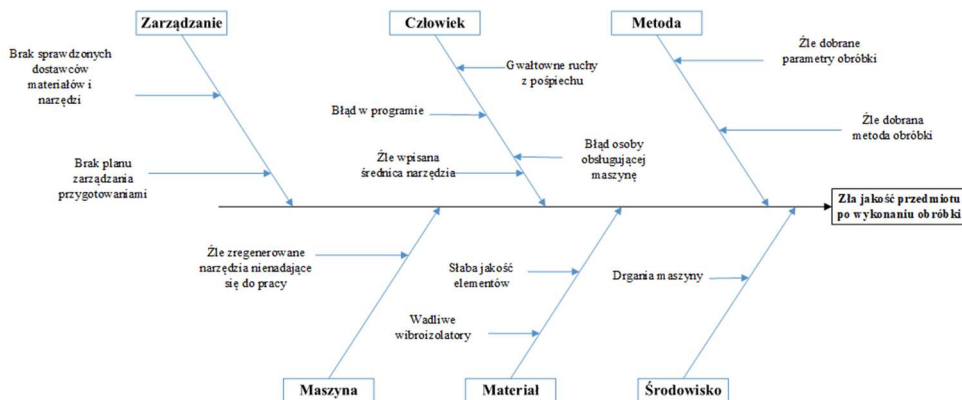
Rys. P15.3. Diagram Ishikawy dla problemu: zła jakość przedmiotu po wykonaniu obróbki Źródło: Opracowanie własne.
